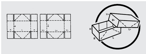
fefco 0304 Stülpkarton, gestanzt mit 4-Punkt-Klebung, Innenfaltung
