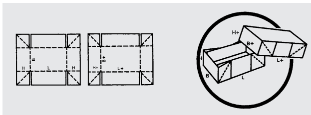
fefco 0308 Stülpkarton, gestanzt mit 4-Punkt-Klebung, Außenklebung
