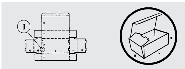
fefco 0421 Wellkartonsschachtel gestanzt, stirnseitig eingeschlagen, mit anhängendem Deckel
