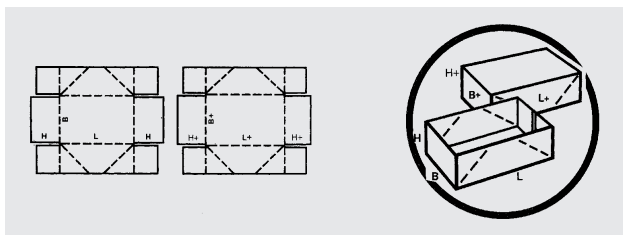
fefco 0303 Stülpkarton gestanzt mit 4-Punkt-Klebung Außenfaltung
