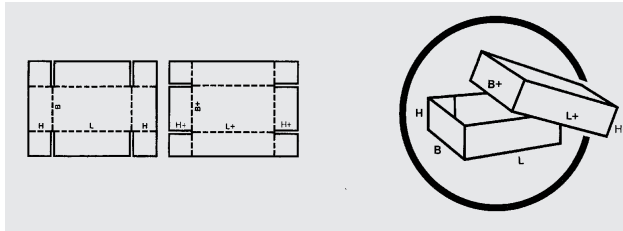
Fefco 301 Stülpkarton, geheftet
