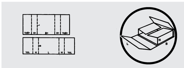
fefco 0404 Kreuzhülle, gerillt
